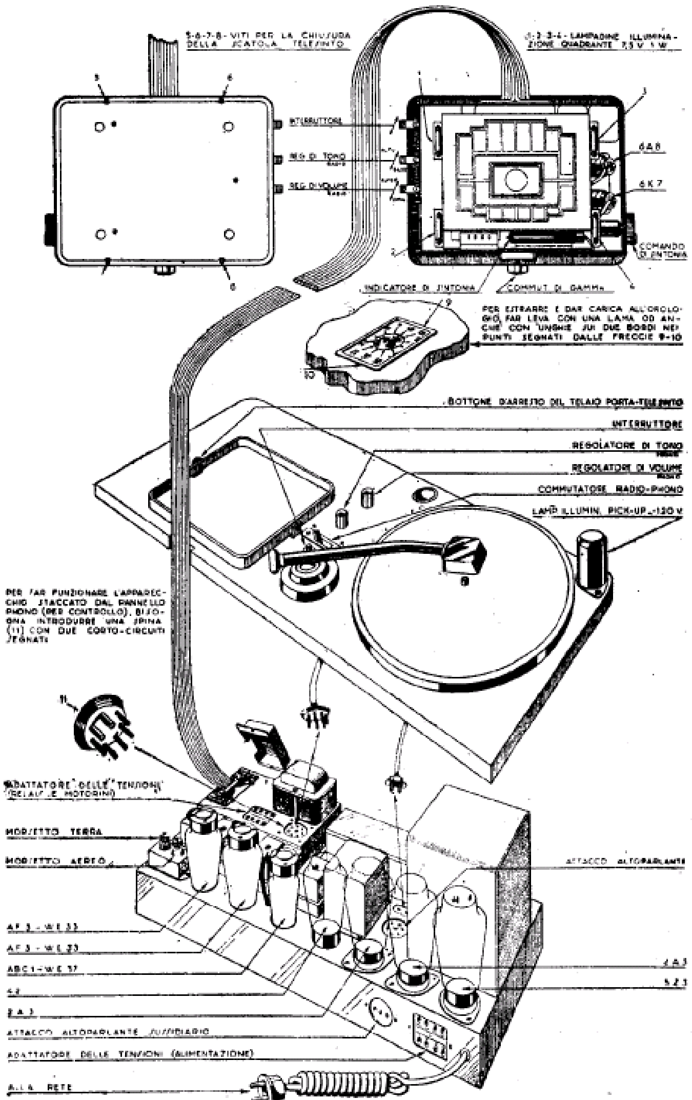
Il piano generale del mod. « 910 » da cui si vede l'esecuzione meccanica del telefinto.
